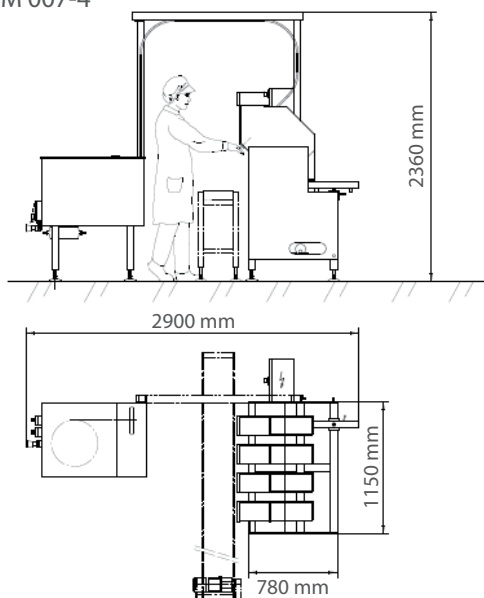
Чертеж BFM 007-4
